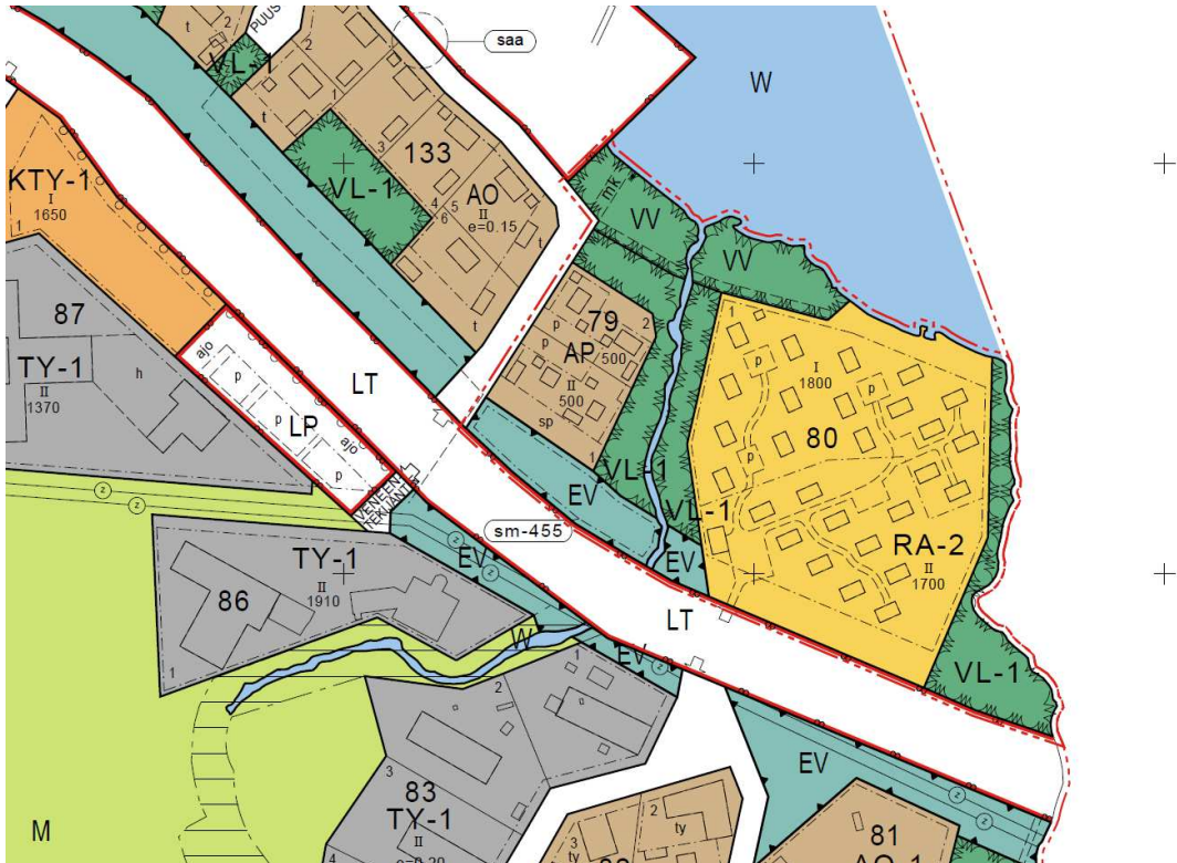
Kuva 4 Ote asemakaavasta.
